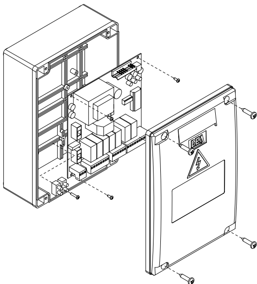
cod. 677050 centrale di comando - art. 202E/3 control board - art. 202E/3 armoire de commande - art. 202E/3 central de mando - art. 202E/3 quadro de comando - art. 202E/3
