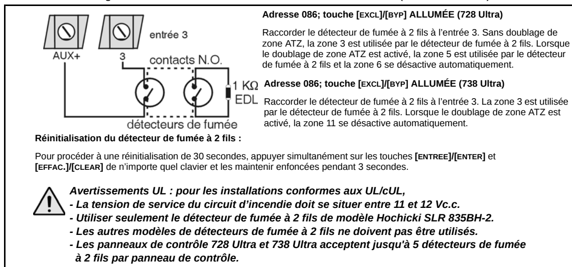
Figure 18 : Raccordement du détecteur de fumée à 2 fils (zone d'incendie)
