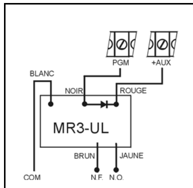
Figure 14 : Relais de la sortie PGM
