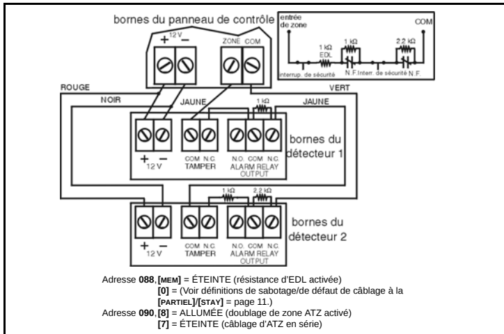
Figure 10 : Contacts N.F., avec résistance d'EDL, reconnaissance de sabotage et de défaut de câblage (UL/cUL)
