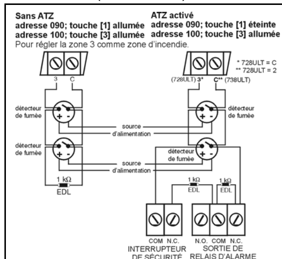
Figure 18 : Raccordement du détecteur de fumée à 2 fils (zone d'incendie)
