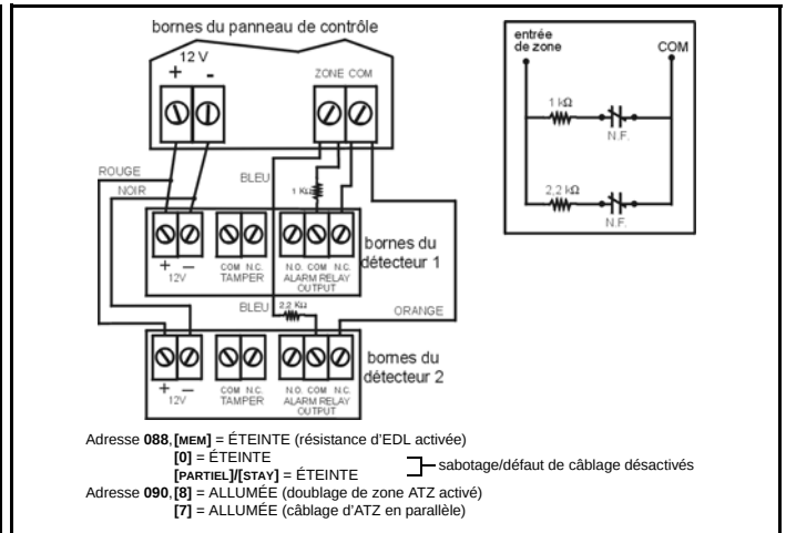
Figure 11 : Câblage en parallèle
