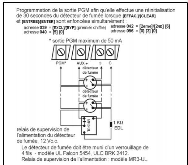
Figure 17 : Réinitialisation du détecteur de fumée à 4 fils
