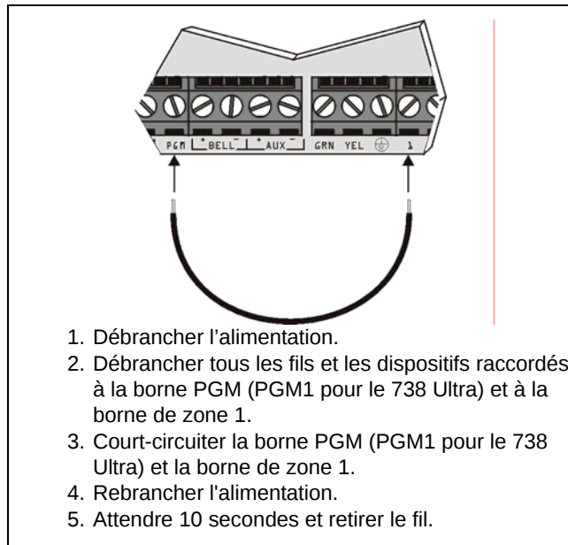
Figure 19 : Réinitialisation par mise hors tension pour le 728 Ultra et le 738 Ultra
