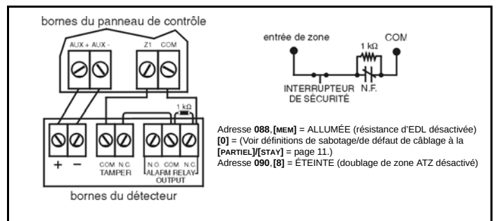
Figure 6 : Contacts N.F., sans résistance d'EDL, avec reconnaissance de sabotage
