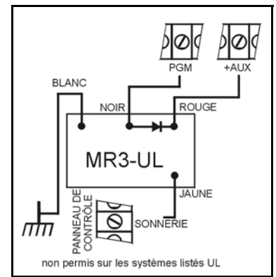
Figure 15 : Circuit de mise en marche par prise de terre
