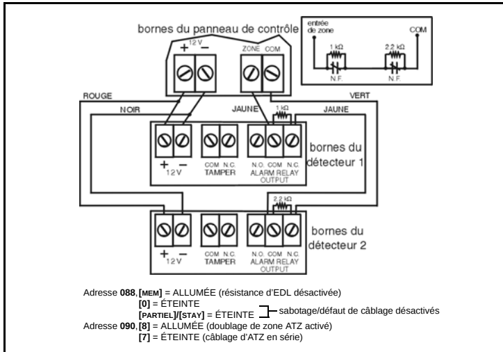
Figure 10 : Contacts N.F., avec résistance d'EDL, reconnaissance de sabotage et de défaut de câblage (UL/cUL)
