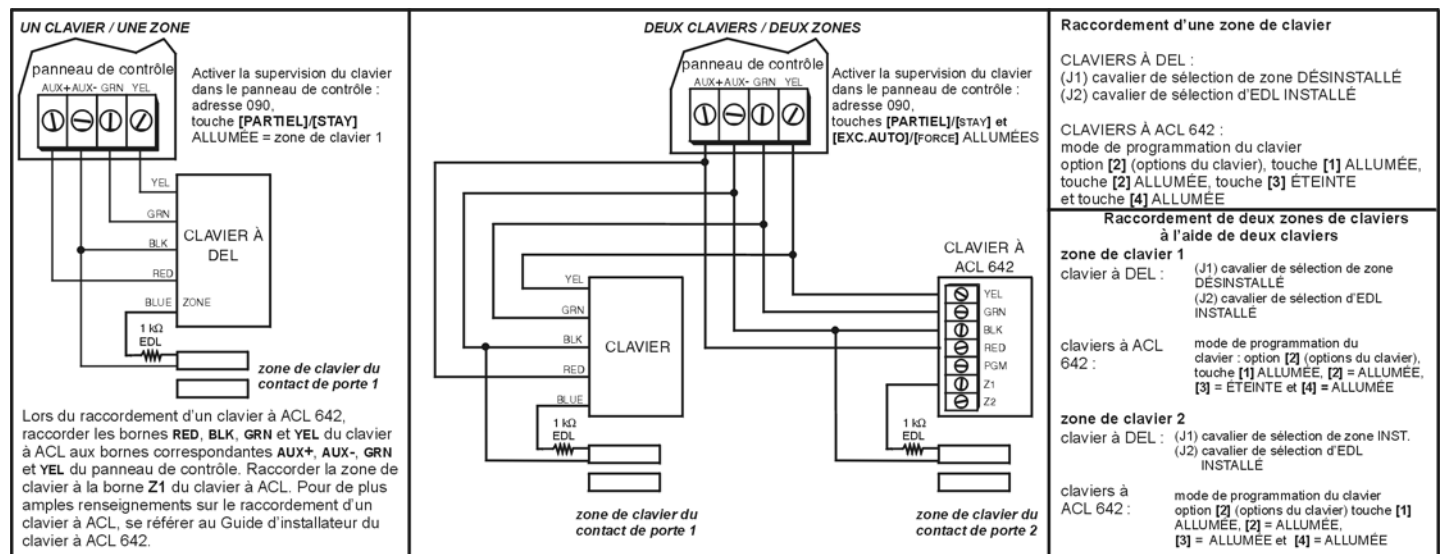
Figure 12 : Raccordement de zones de clavier
