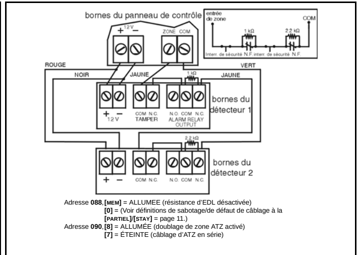
Figure 11 : Câblage en parallèle
