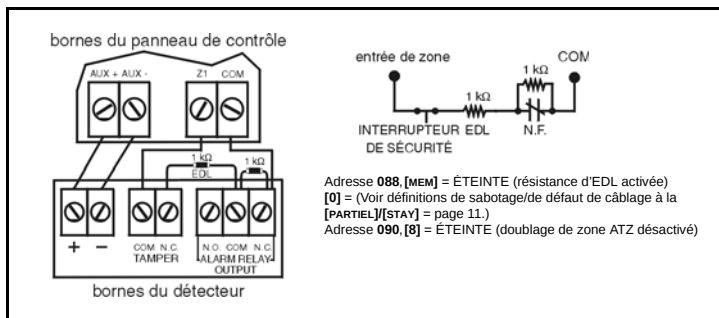
Figure 7 : Contacts N.F., avec résistance d'EDL, reconnaissance de sabotage et de défaut de câblage (UL/cUL)
