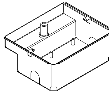
cod. 386180 cassa di fondazione inox stainless steel foundation box caisson inox
