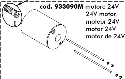
cod. 923180U vite senza fine+spina worm screw+pin vis sans fin+goupille tornillo sinfin+clavija parafuso sem fin+ficha
