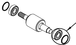
cod. 933060G albero motore - non rev. motor shaft - not rev. arbre moteur - non rev. eje motor - no rev. veio do motor - não rev.
