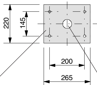
Base di ancoraggio armadio Mounting base for case Base d'ancrage armoire Ankerplatte Schrank Base de anclaje armario
