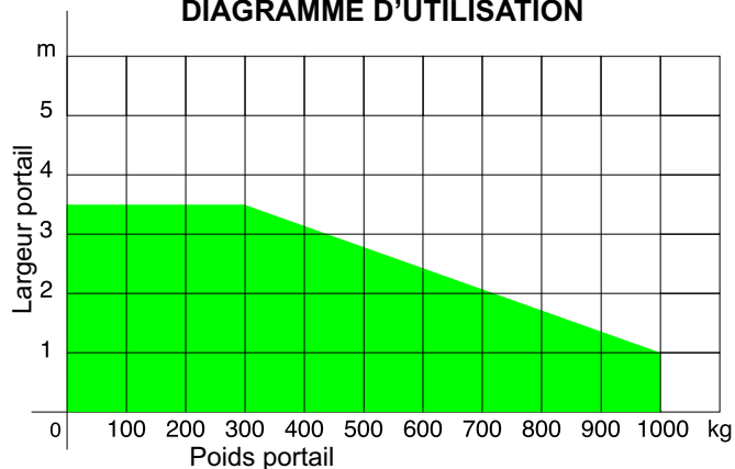
DIAGRAMME D'UTILISATION
